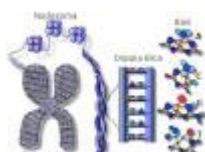
dna_structure.jpg
